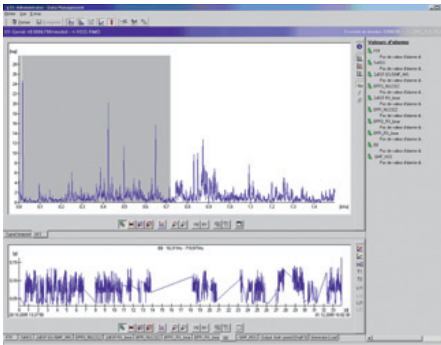
Surveillance d'une bande large
